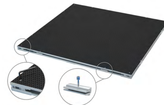
Mâchoires et fixations
